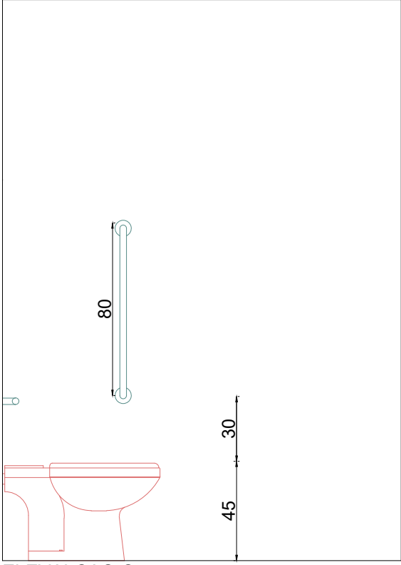
ELEVALÇÃO C
