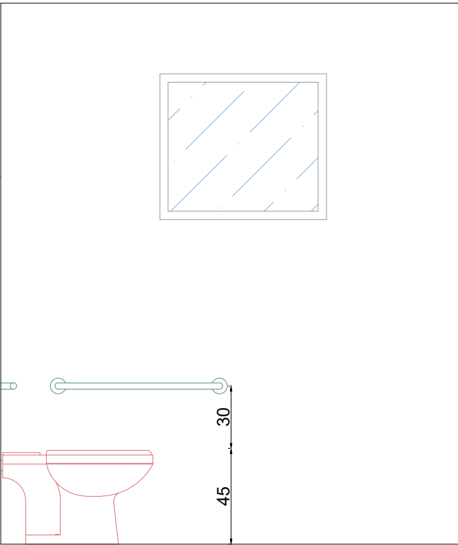
ELEVALÇÃO B
