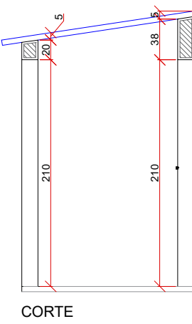
CORTE
