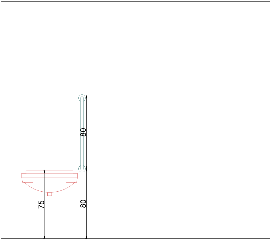
ELEVALÇÃO A
