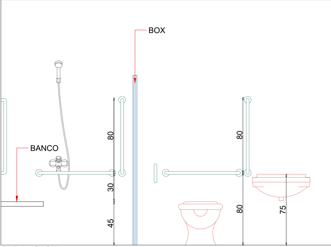
ELEVALÇÃO B
