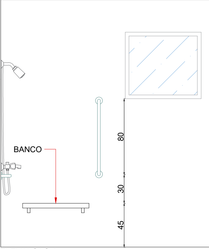
ELEVALÇÃO A
